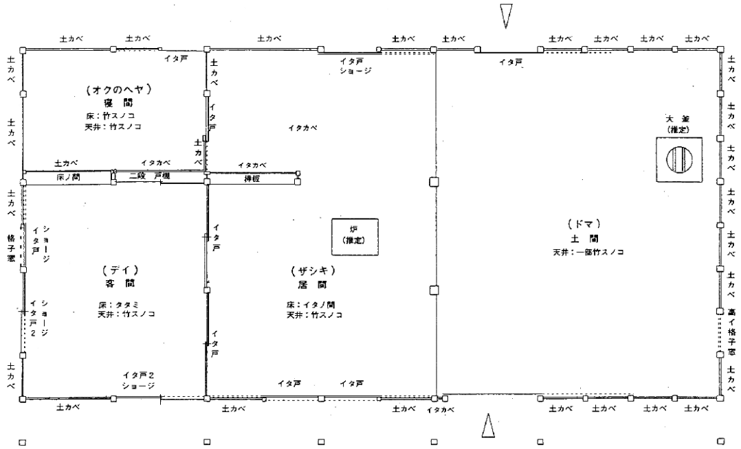
旧高橋家住宅 復元平面図
