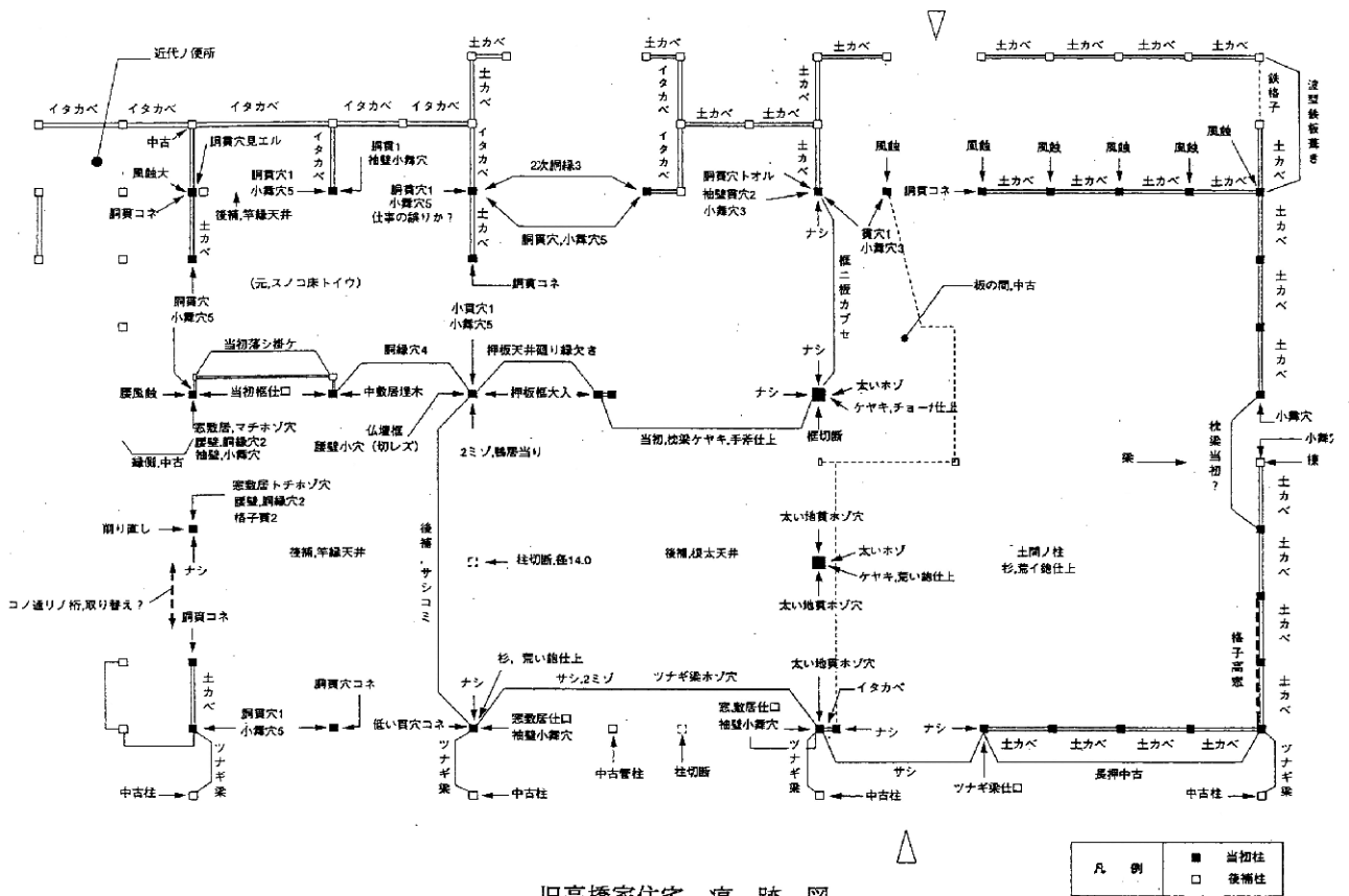
旧高橋家住宅 痕跡図
