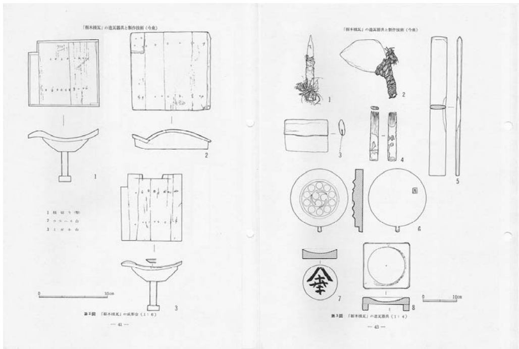
榎木棧瓦の製作用具（今泉1984より）
