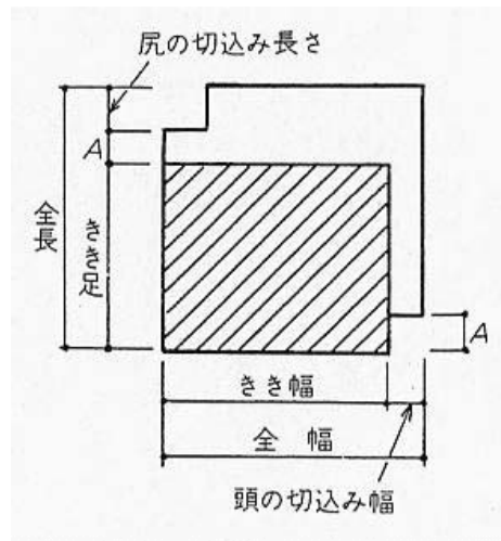
棧瓦の葺き足（坪井1977年より）
