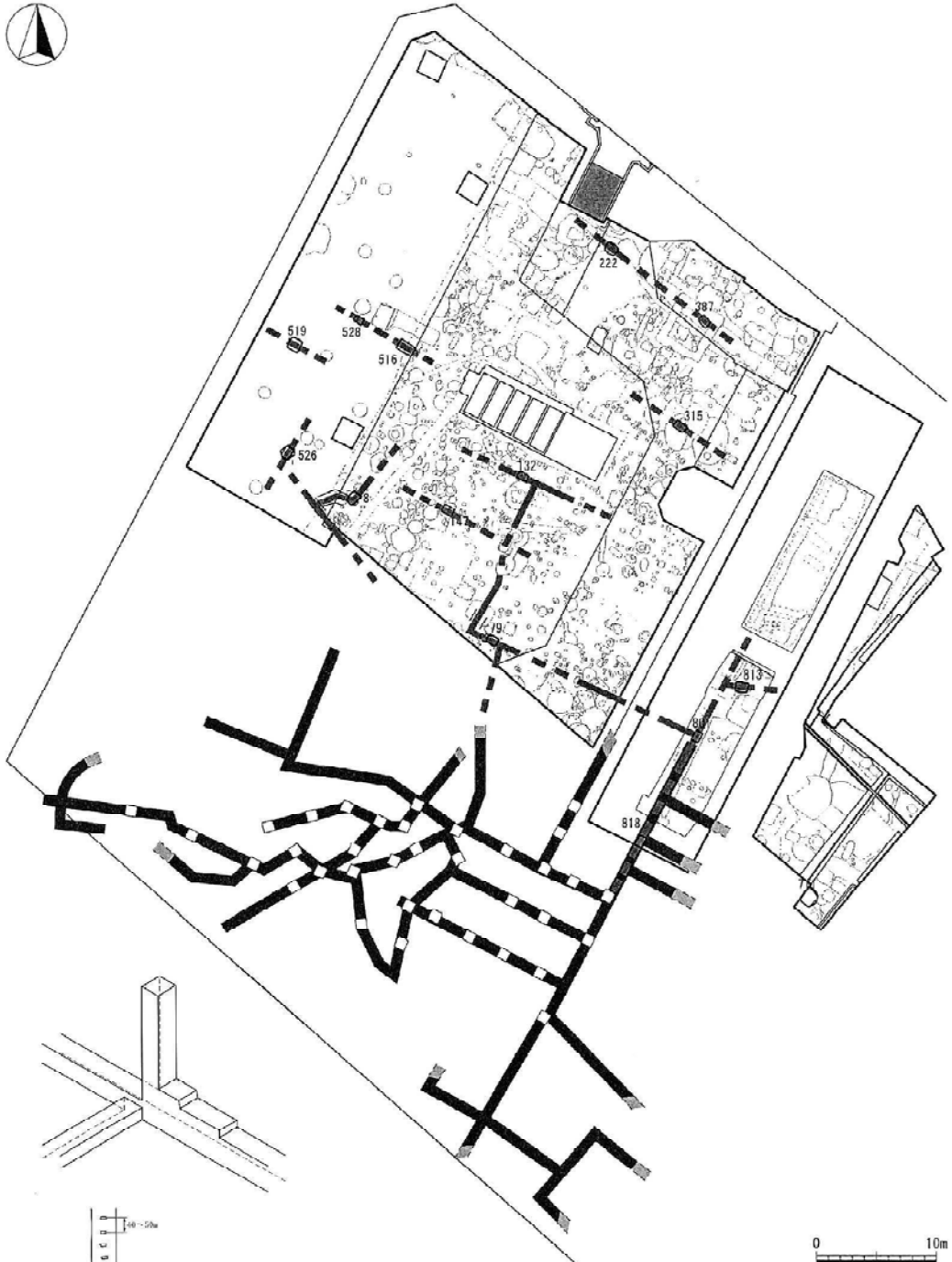
第6図 大塚窪町遺跡地下坑平面図
