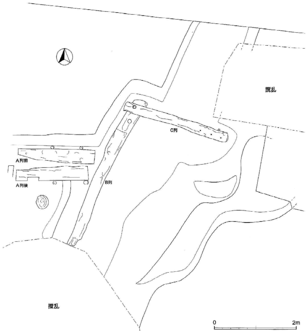
第21図 石垣下胴木平面図
