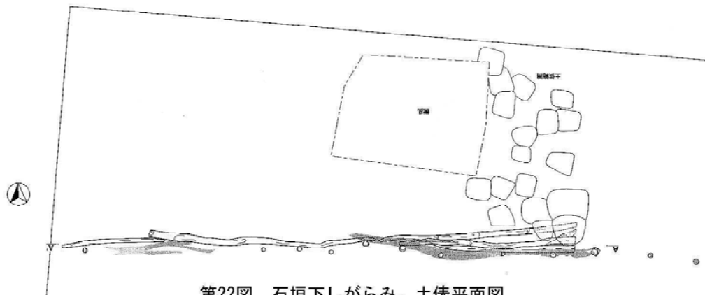
第22図 石垣下しがらみ。土俵平面図
