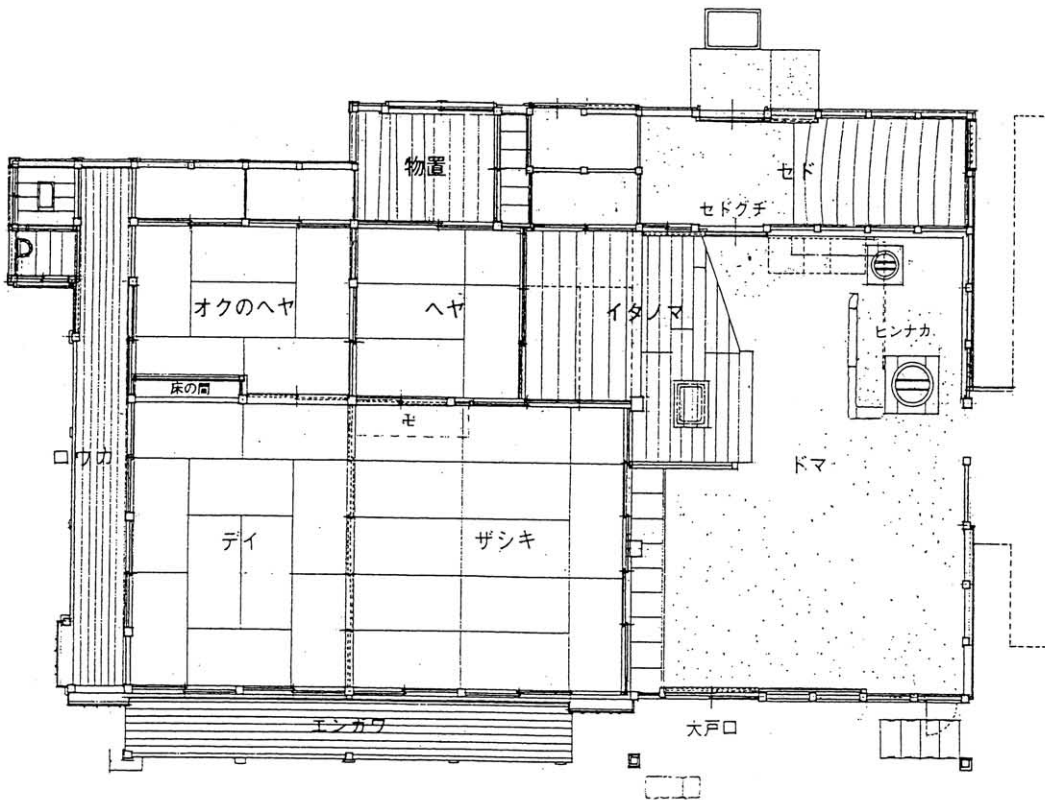
旧高橋家住宅 現状平面図
