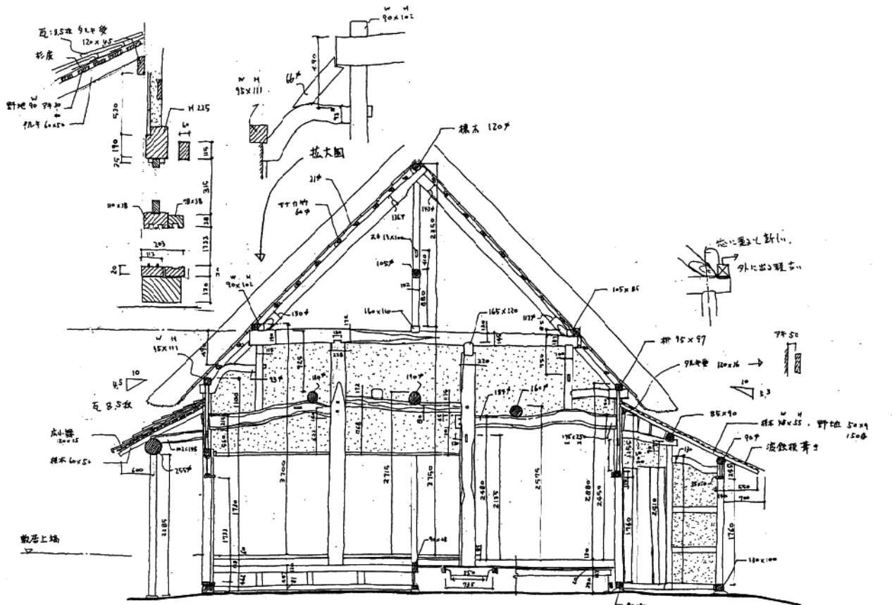
(朝霞)旧高橋家 断面図 I '10.12.18,25 大ヒラ
